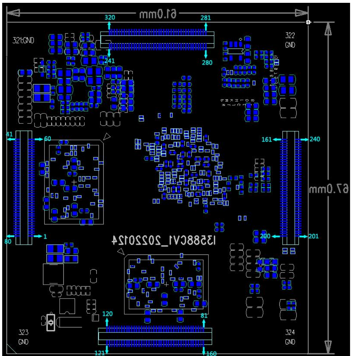
BOT 层
