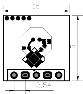
图 5 参考尺寸(15mm*15mm*2mm)
