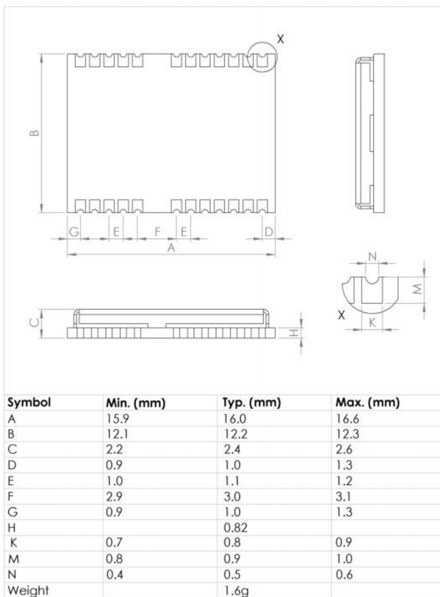
图 3 尺寸图
