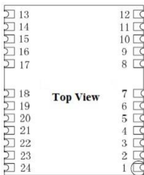
图 2 引脚分布图
