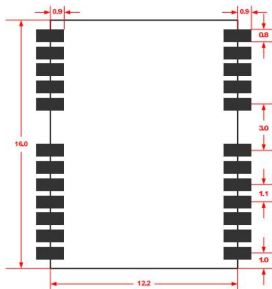
图 7 CNT216A 封装参考
